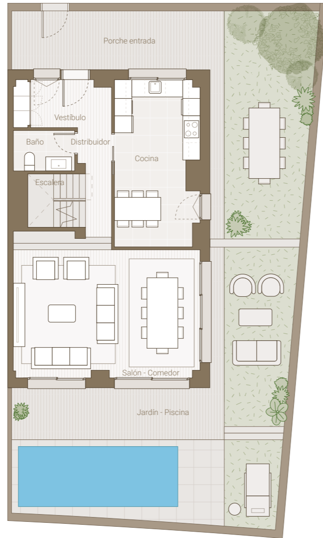
PLANTA BAJA
